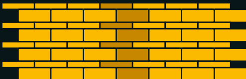
Läuferverband mit Rollschicht
