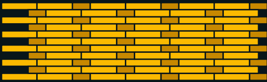
Läuferverband halber Stein versetzt
